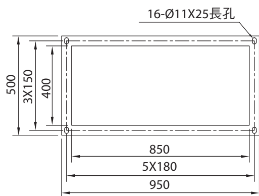
12kV級導口
