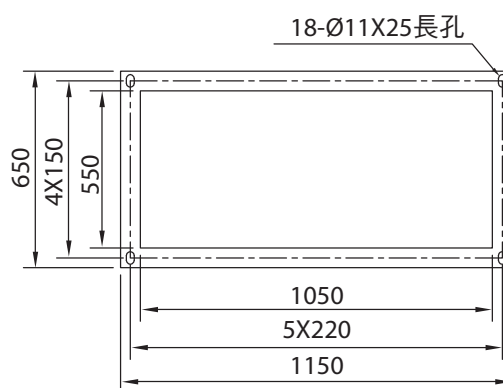
24kV級導口
