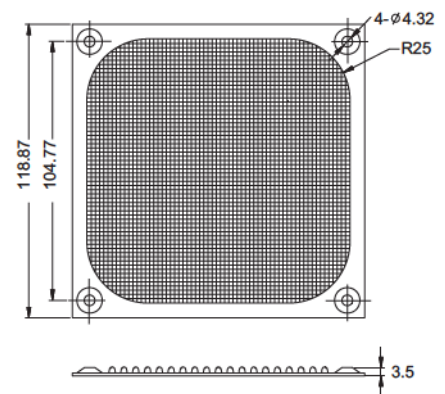
FM 12 For 120mm Fan
