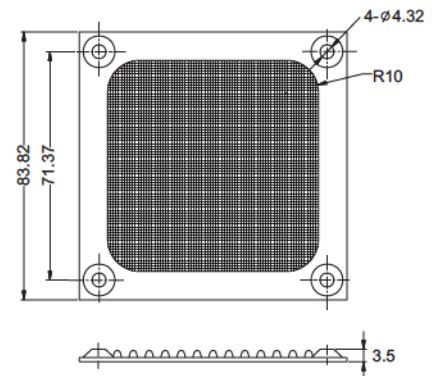
FM 08 For 80mm Fan
