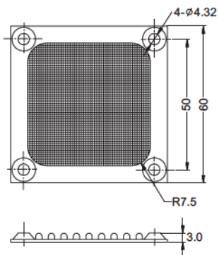
FM 06 For 60mm Fan
