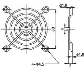
FG-06 For 60mm Fan
