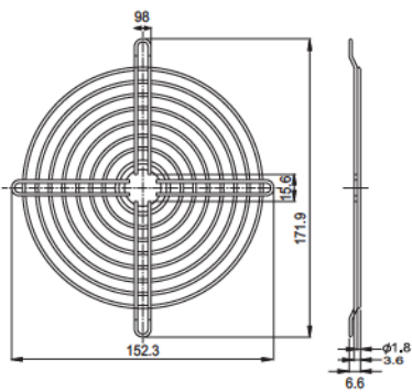
FG-18B For 176mm Fan
