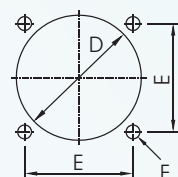
門板鑽孔圖
